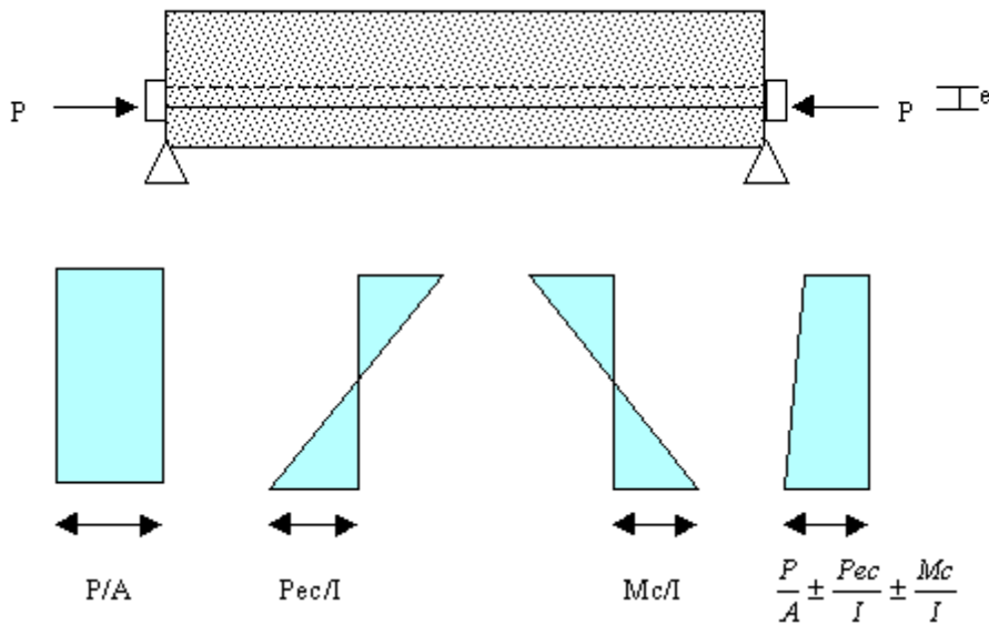
Figura 2. Distribución de esfuerzo a través de una sección de concreto presforzado excéntricamente
