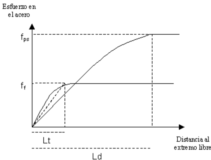
Figura 3.1. Longitudes de transferencia y desarrollo para cables de pretensado.
