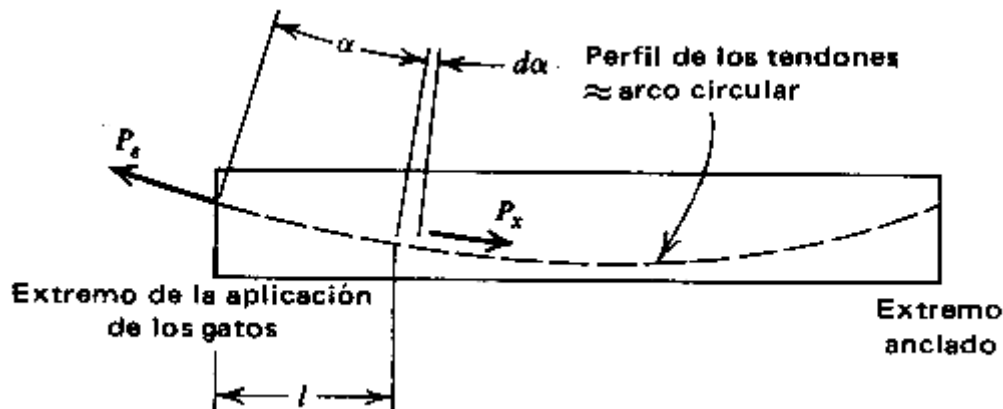
Figura 2.1. Pérdida de presfuerzo debida a la fricción por curvatura.
