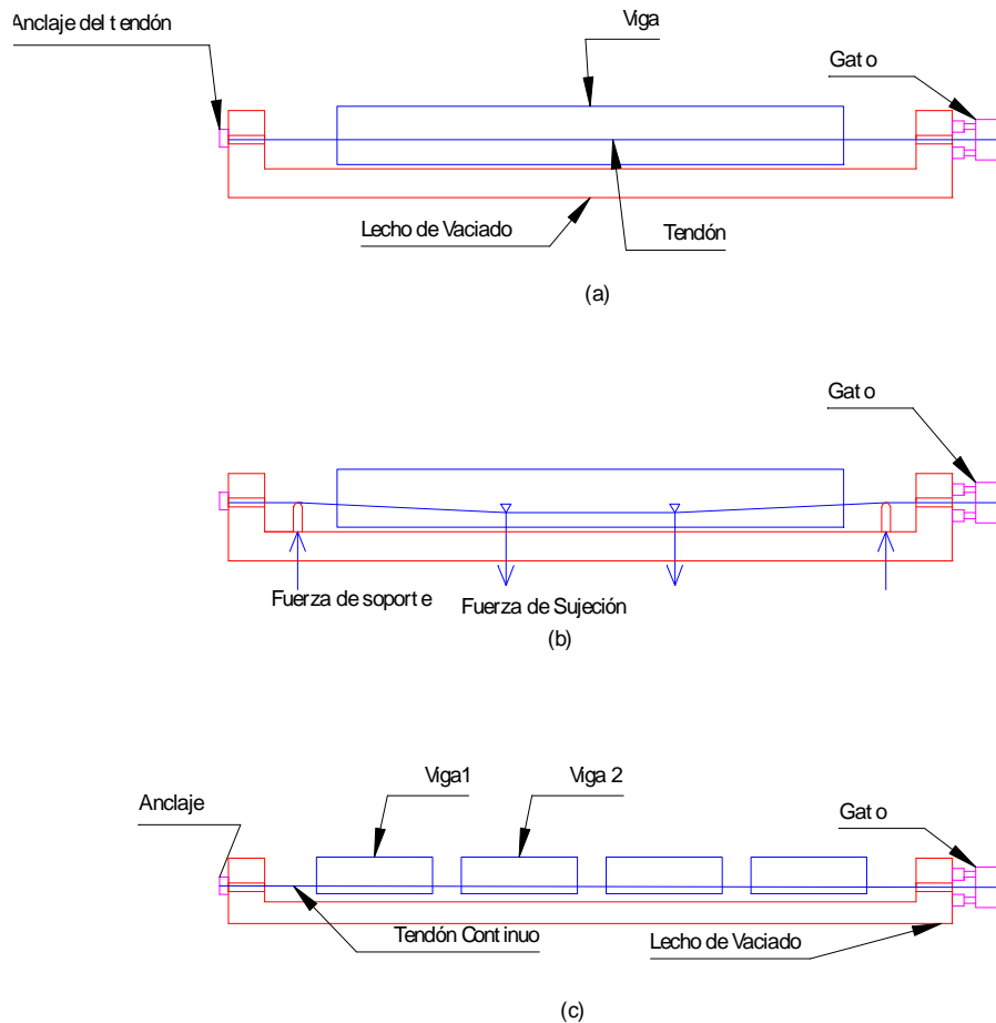
Fig.1.3 Métodos de pretensado. a) Viga con tendón recto. b) Viga con excentricidad variable del tendón. c) Esforzado y vaciado de línea larga
