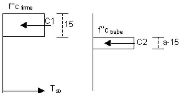
Figura 4.1. Diagrama de esfuerzos.
