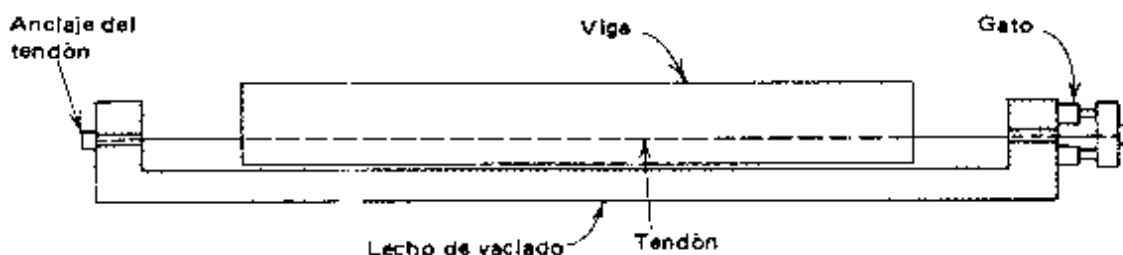
Figura 6. Fabricación de un elemento pretensado
