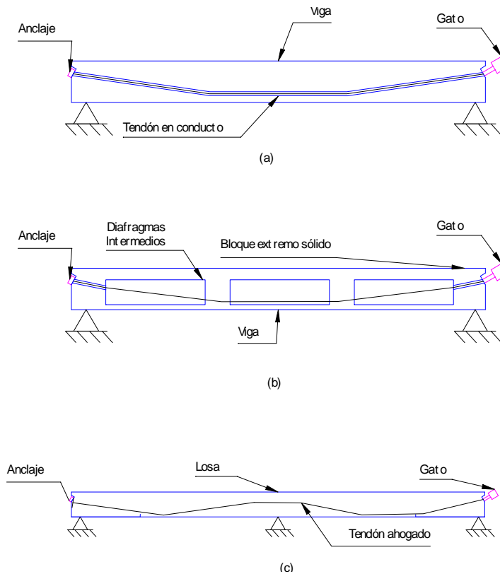
Fig. 1.4 Métodos de postensado a) Viga con conducto hueco embebido en el concreto. b) Viga celular hueca con diafragmas intermedios. c) Losa continua con tendones envueltos, revestidos con asfalto.
