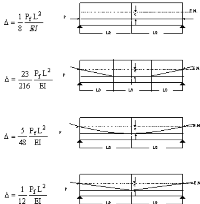
Figura 3.5 .Deflexiones al centro del claro para algunos tipos de elementos pretensados simplemente apoyados. (Referencia 13)
