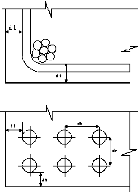
Figura 3.6 - Recubrimiento y separación libre de varillas y torones
