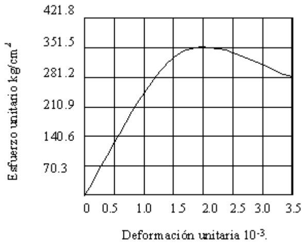
Figura 8. Curva típica esfuerzo-deformación para concreto de 350 kg/cm 2 .
