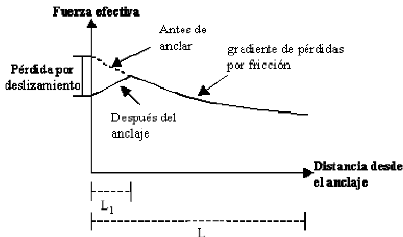
(a) Tensando de un lado
